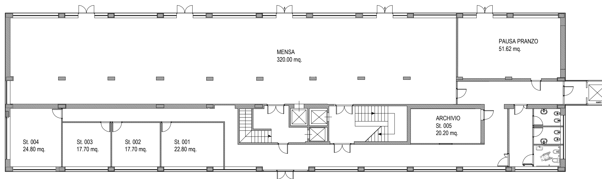
PALAZZINA D PIANTA PIANO PRIMO INTERRATO Q. -3.50 (680 MQ.) 1:200
